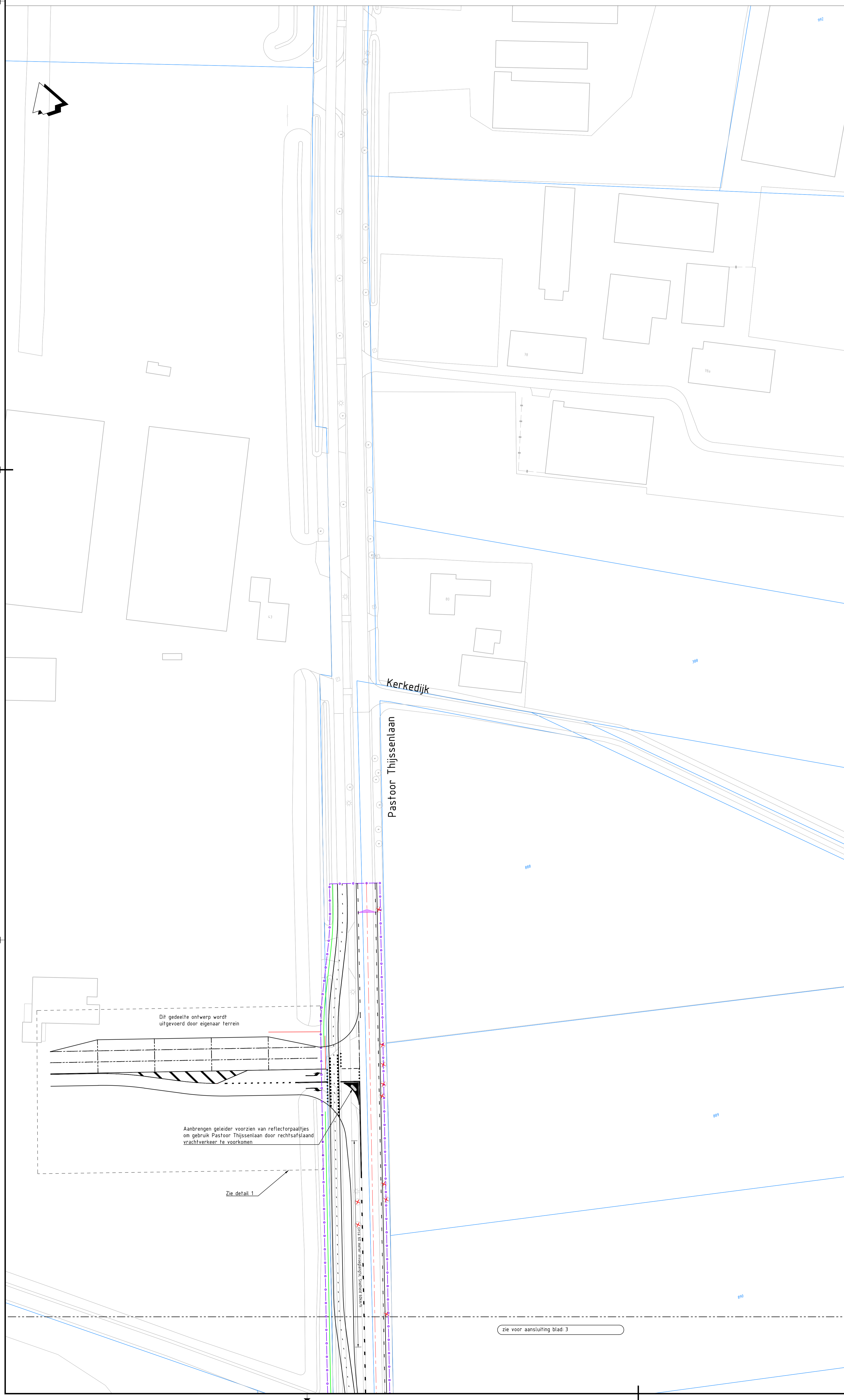
DETAIL 1 Herinrichtingsvoorstel entree Bedrijventerrein met uitgebogen wijzigend fietspad en voorangsregeling schaal 1:250
